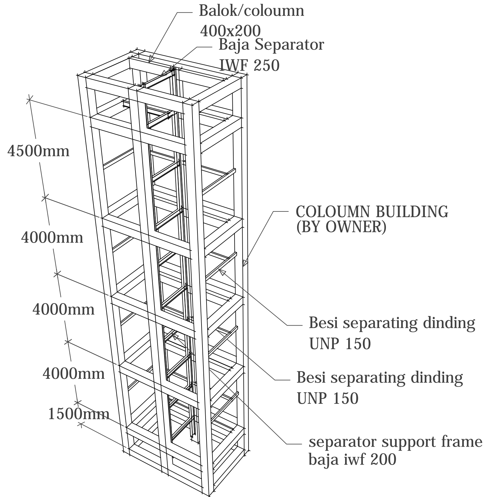
ISOMETRIC TAMPAK DEPAN
